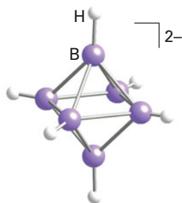
5 [\text{B}_6\text{H}_6]^{2-}
