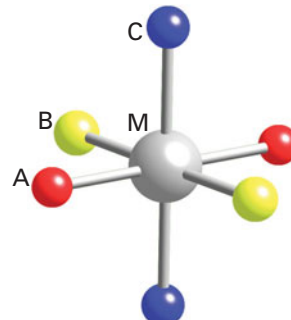
58 [MA 2 B 2 C 2 ]
