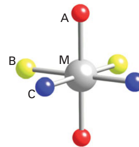
59 [MA 2 B 2 C 2 ]
