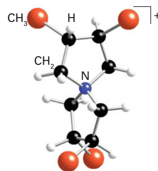
12 [N(CH_2CH(CH_3)CH(CH_3)CH_2)_2]^+
