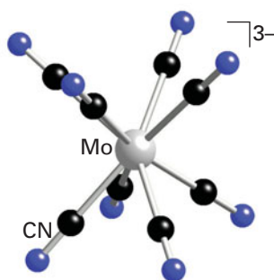
28 [Mo(CN) 8 ] 3- ( D_4 )
