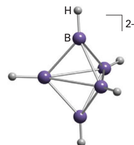
4 [\text{B}_5\text{H}_5]^{2-}
