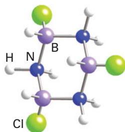
25 B_3N_3H_3Cl_3
