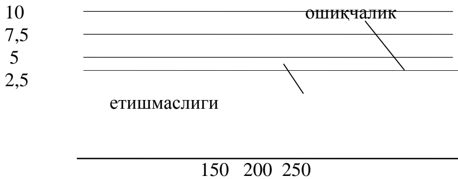
2.5.1-чизма. Пул бозорида тенгликга эришиш.
