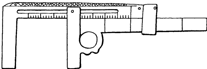
Рис. 77. Измерительный прибор с нониусом, позволявший проводить измерения с точностью до \frac{1}{10} дюйма (2 мм); на оборотной стороне — дата изготовления: 15 января 9 года н. э. Шанхай
