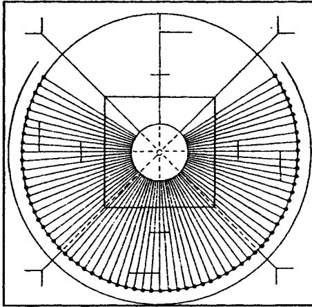
Рис. 25. Солнечные часы (реконструкция)
