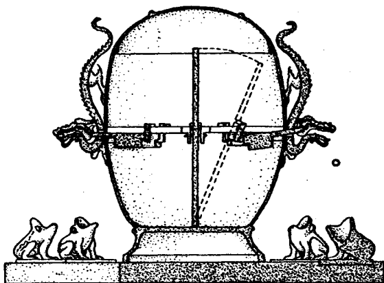
Рис. 27. Тот же прибор в разрезе
