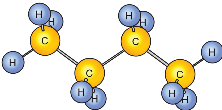
Kimyoviy bog'lanish xarakteristikasi
