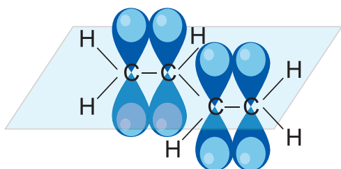
p -elektron buluti
