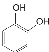
pirokateksin (benzendiol-1,2; 1,2-digidroksi- benzol)
