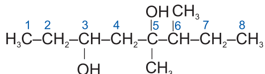
propan triol -1,2,3 (glitserin)
