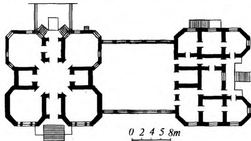
Qo'qon. Rus-Osiyo banki, 1910-y arxitektor I. Markevich. Umumiy ko'rinishi va tarhi (M. Yusupova kitobidan).
