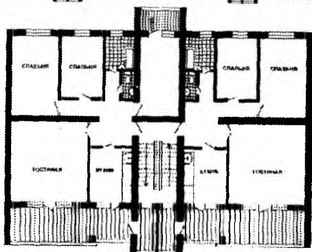
Toshkent. Qunayev ko'chasidagi yanada yaxshilangan rejali turar-joy majmui. «Toshgiprogor» instituti.
