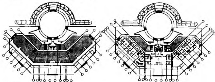
Qarshi. Amfiteatr, 2006-y. Arxitektorlar S. Sutyagin, A. Zohidov. Umumiy ko‘rinishi, birinchi va ikkinchi qavat tarhlari.
