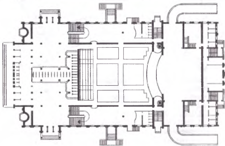
Temiryolchilar Madaniyat saroyi, 1939-y, arxitektor A.Pavlov. Umumiy ko'rinishi va birinchi qavat tarxi.
