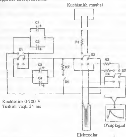
2.12-rasm. Elektroporatsiyani amalga oshirish uchun past kuchlanishli qurilmaning tuzilishi.
