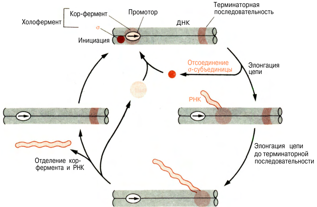
РИС. 3.5. «Рабочий цикл» \sigma -субъединицы. Кор-фермент связывается с \sigma -субъединицей, образуя холофермент, который прочно связывается с промотором. После запуска
