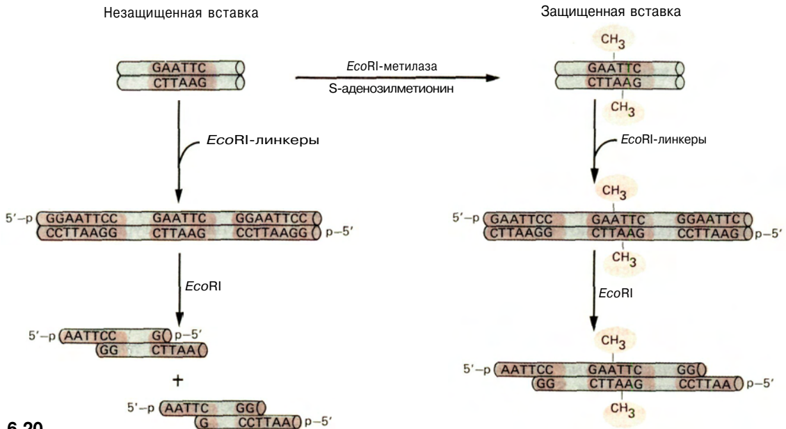
РИС. 6.20. Сайты для рестриктирующей эндонуклеазы, находящиеся во встроеном фрагменте, защищены путем мети-
