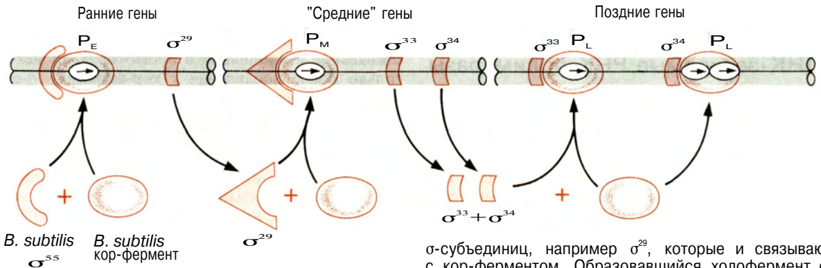
РИС. 3.6. Схема, иллюстрирующая участие различных \sigma -субъединиц в споруляции у B. subtilis . Некоторые \sigma -субъединицы, в частности \sigma^{55} , присутствуют и в вегетативных клетках. В условиях, стимулирующих споруляцию (в частности, голодание), появляется несколько новых
