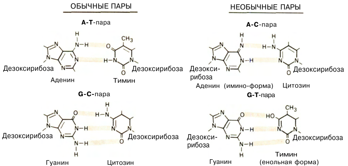
РИС. 2.14. Сравнение обычных и необычных, редко встречающихся пар оснований.
