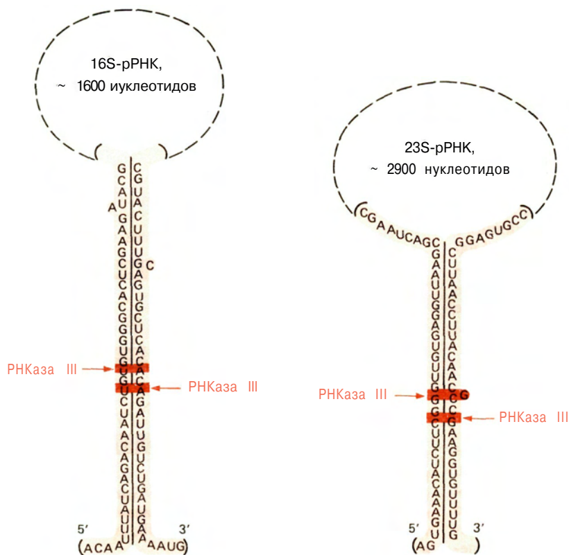
РИС. 3.15. Сайты расщепления для РНКазы III в предшественниках рРНК. Эти сайты находятся в стебле, образуемом при внутримолекулярном спаривании оснований спейсерных участков, фланкирующих 16S- и 23S-рРНК-последовательности. [B. Lewin, Genes III (New York: Wiley, 1987), p. 453.]
