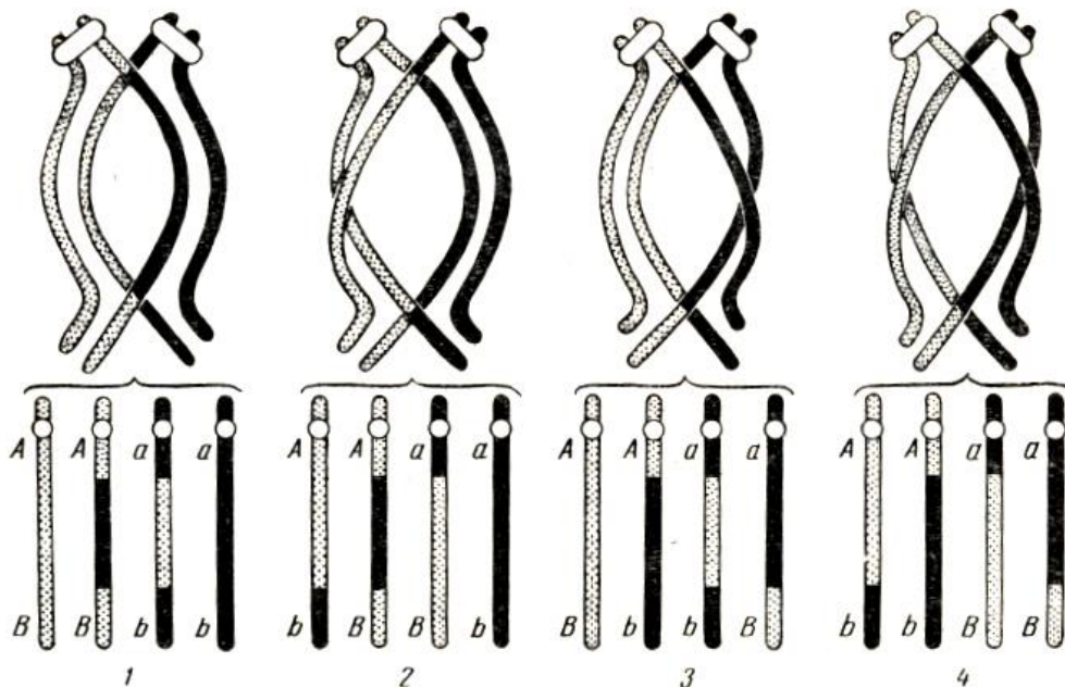
50-расм. Якка кроссинговердан сўнг гаметаларнинг ҳосил бўлиши. 1 - ота-она генларига ўхшаш гаметалар; 2 - рекомбинант генли гаметалар.
