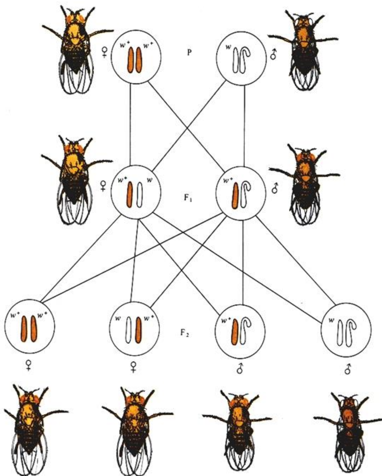
44.1-расм. Drosophila melanogaster да жинс билан бириккан ҳолда ирсийланиш. Қизил кўзли урғочи пашшалар ва оқ кўзли эркак пашшалар ўзаро чаштирилган. w^+ ва w символлари билан мос равишда қизил кўзли ва оқ кўзли аллеллари белгиланган.
