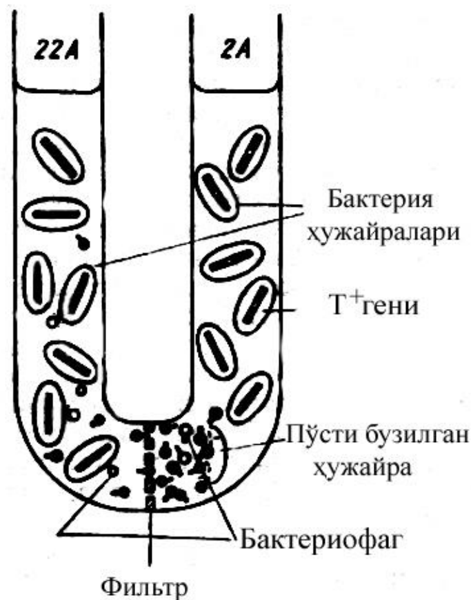
67-расм. Salmonella typhimurium бактериясида трансдукция ходисасини кўрсатувчи тажриба схемаси. 22А бактерия штамлари триптофанны синтез қила олмайди ( T^- ), 2А - триптофанны синтезловчи ( T^+ ) штамм.
