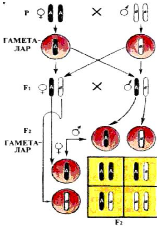
10-расм. Монодурагай чатиштиришдаги ирсийланишнинг цитологик асослари.
