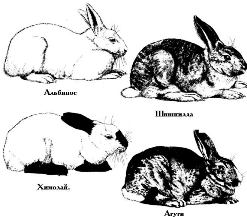
13-расм. Қуёнларда жун рангининг ирсийланиши.
