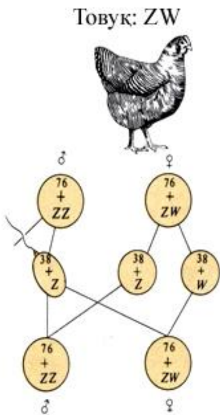
43-расм. Жинси белгилашнинг тўртта типи.
