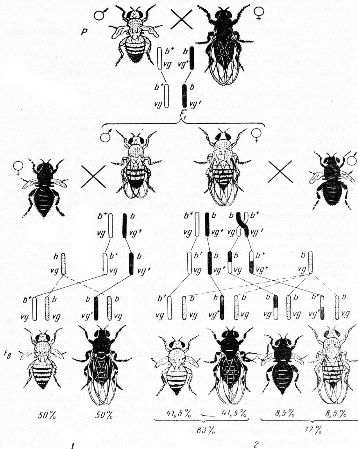
46-рasm. Дрозофилада белгиларнинг бириккан ҳолда ирсийланиши. 1-кроссинговер кузатилмаган ҳолат (F 1 нинг гетерозиготали эркак пашшаси); 2- кроссинговер рўй берган ҳолат (F 1 нинг гетерозиготали урғочи пашшаси). F B да фақат урғочи пашшалар.
