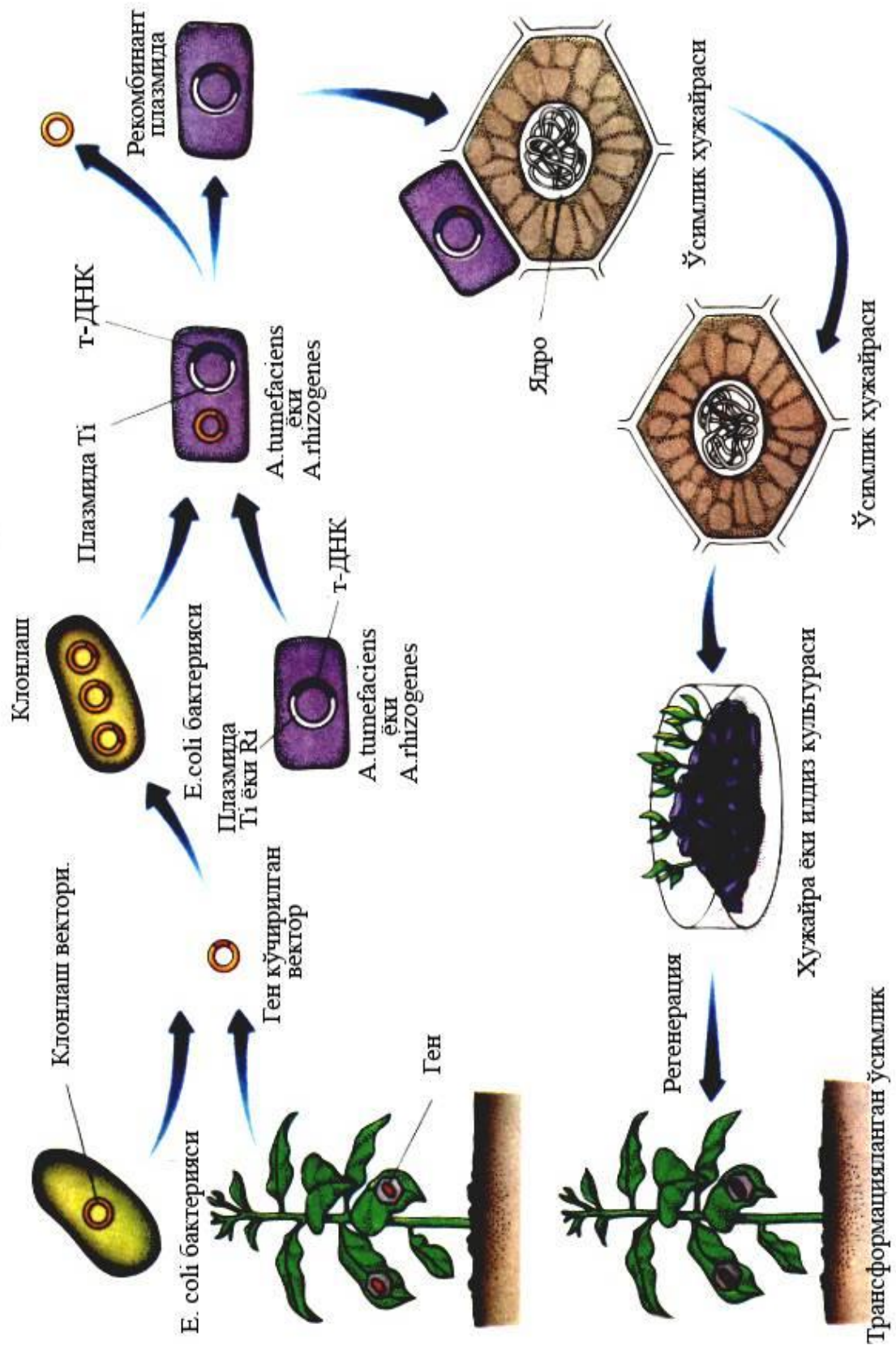
92-расм. Ўсимликларда ген инженерияси методи қўлланиш механизмининг схемаси
