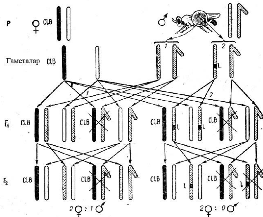
98-расм. Дрозофилада жинс билан бириккан рецессив летал мутацияларни аниқлашнинг CIB методи.
