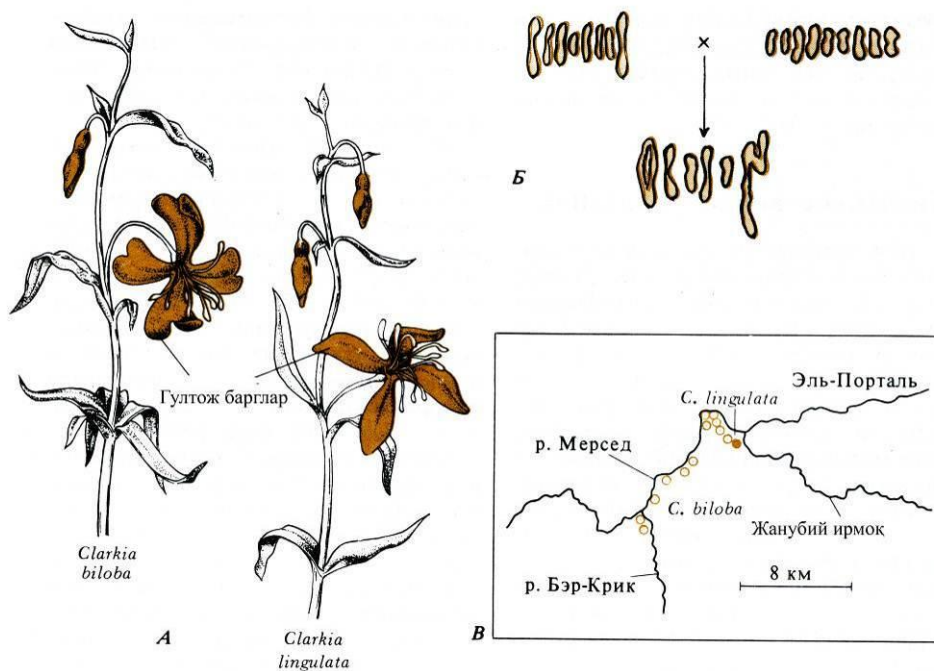
122-расм. Бир йиллик ўсимликларнинг икки тури.
