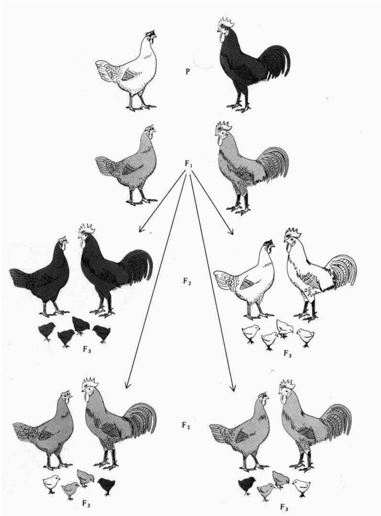
5-расм. Андалузия товукларида пат рангининг ирсийланиши.
