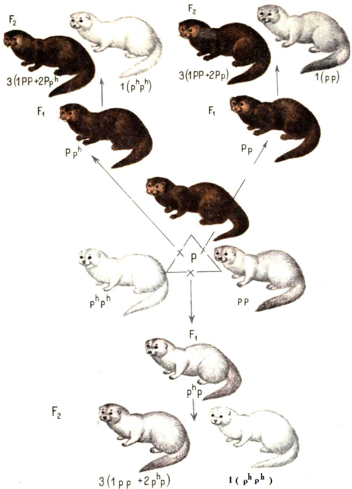
14-расм. Қоракузанларда мўйна рангининг ирсийланиши. Р-жигар рангли (ёввойи тип); р- платина рангли; р h -оқ рангли.
