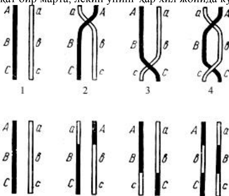
49-расм. Кўш кроссинговернинг соддалаштирилган схемаси.
