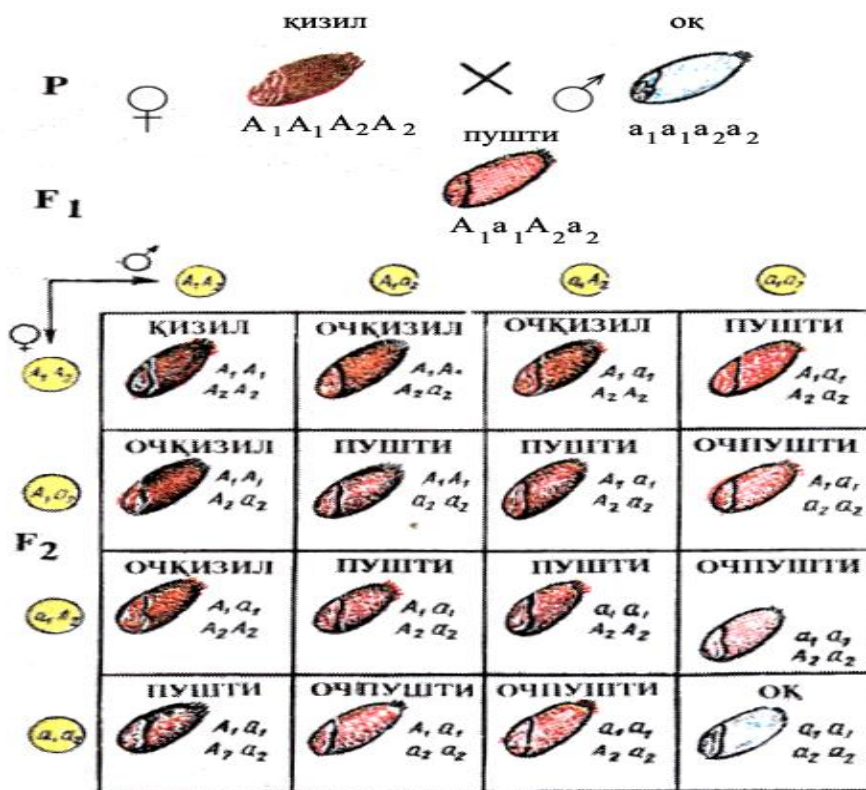
21-расм. Генларнинг полимер таъсирида бугдой дони рангининг ирсийланиши.
