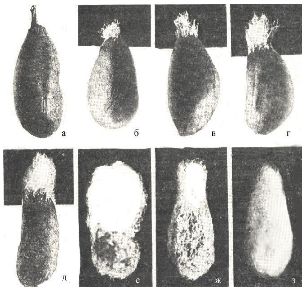
30-расм. G.hirsutum L. турига мансуб ғўзаларда чигит тукланишининг типлари: а – ГС-яланғоч уруғли; б – н3-МС-жуда кичик микропиляр тукланиш; в – м-МС-ўртача микропиляр тукланиш; г – п-МС-оралиқ микропиляр тукланиш; д – н-МС-нормал микропиляр тукланиш; е – б-МС- катта микропиляр тукланиш; ж – ПС-чигитнинг микропиляр қисмида нормал тукланиш, халаза қисмида тукланишнинг нотекис тақсимланиши; з – ОС-чигитнинг тўлиқ тук билан қопланиши.
