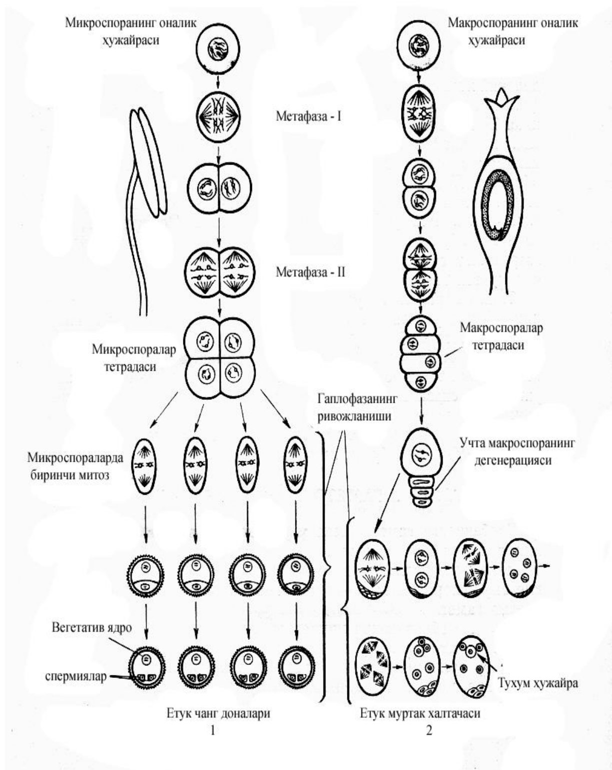
39-расм. Ривожланишнинг қиёсий схемаси. Гулли ўсимликларда эркаклик микроспорогенези ва микрогаметогенези (1), урғочилик макроспорогенези ва макрогаметогенези (2) ҳамда жинсий ҳужайраларнинг етилиши.
