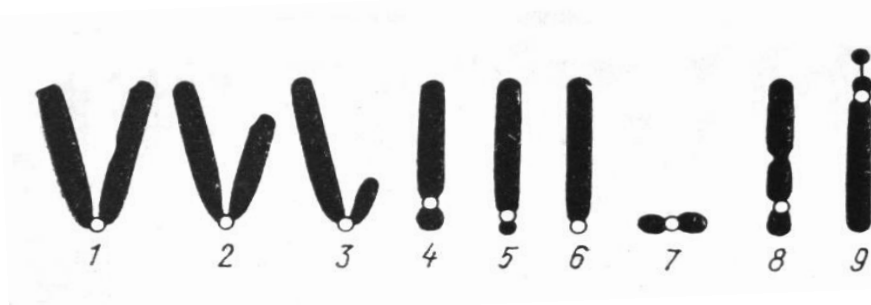
33-расм. Метафаза босқичидаги хромосомаларнинг ҳар хил типлари.
