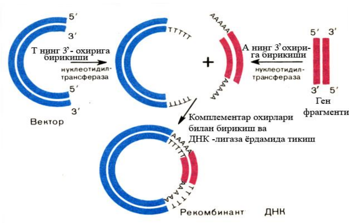
88-расм. Рекомбинант ДНК синтез қилинишининг схемаси.
