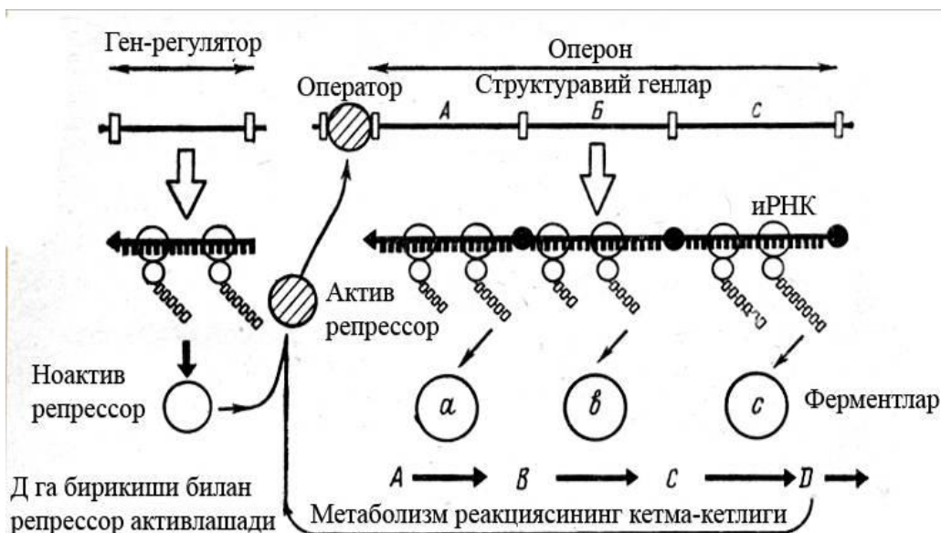
85-расм. Структуривий генлар фаолиятининг бошқарилиши.
