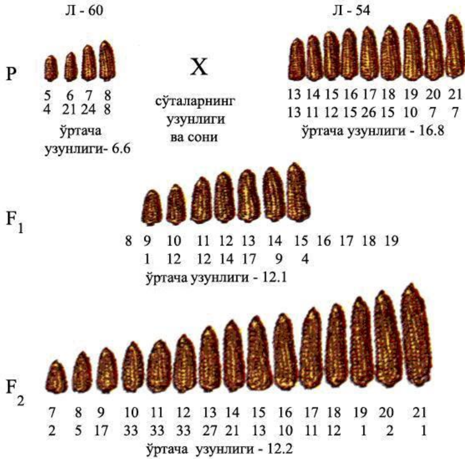
23-расм. Маккажўхорида сўта узудлигининг ирсийланиши (см. ҳисобида).
