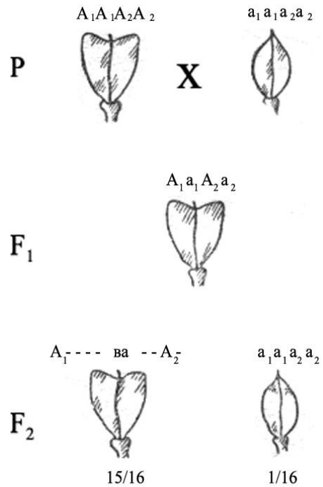
25-расм. Capsella bursa pastaris (ачамбити) ўсимлигида кўзоқ мева шаклининг ирсийланиши.
