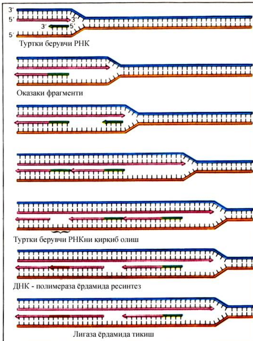
72.2-расм. ДНКнинг 5' -3' ва 3' -5' йўналишдаги нуклеотид занжирларининг репликацияси.
