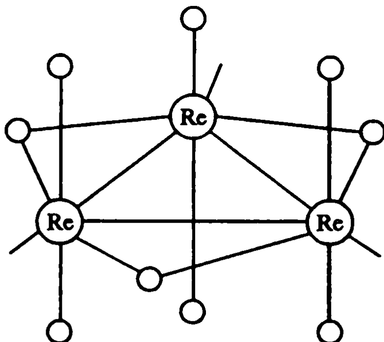
XII.2-расм. [\text{Re}_3\text{Cl}_{12}]^{3-} анионининг фазовий тузилиши.
