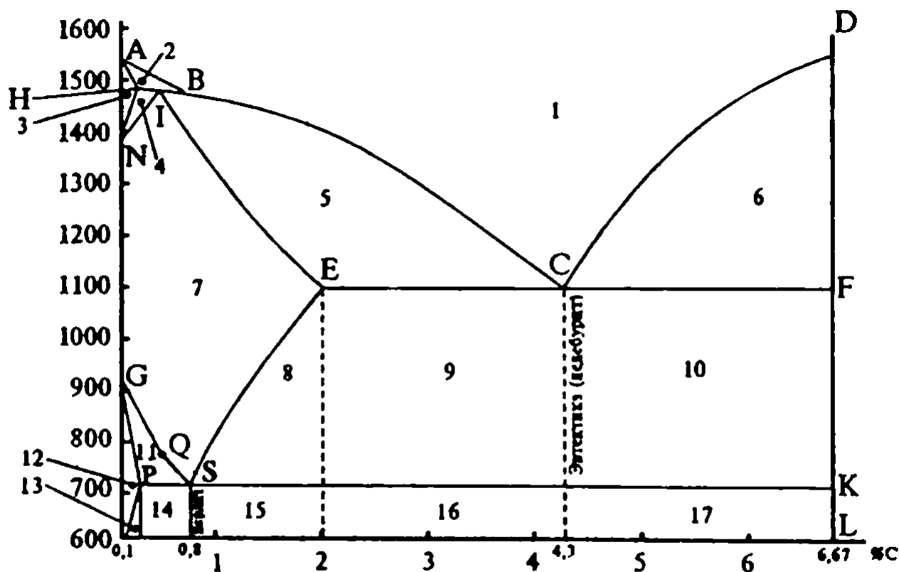
XII.5-расм. Fe — C системанинг ҳолат диаграммаси.
