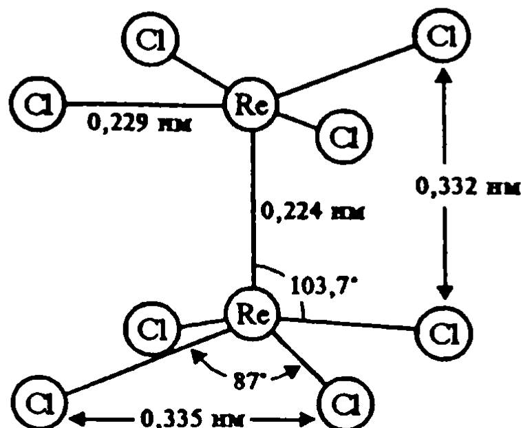
XI.2-расм. [\text{Re}_2\text{Cl}_8]^{2-} анионининг фазовий тузилиши.
