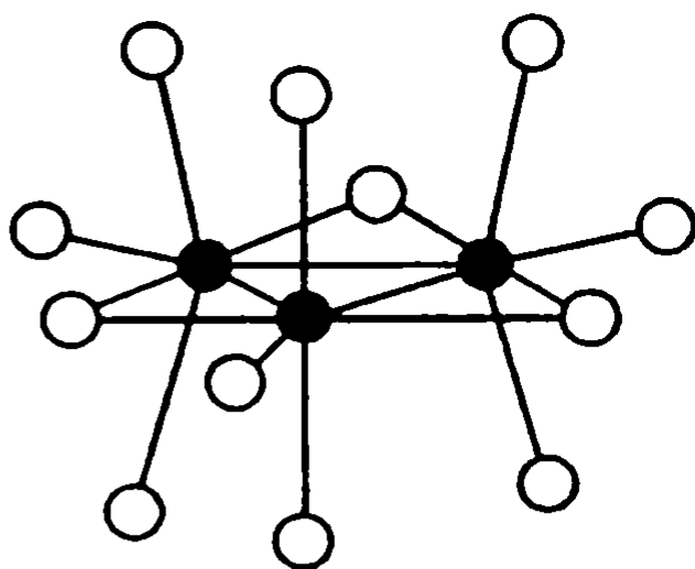
XI.4-расм. Уч ўзакли [Re 3 Cl 12 ] 3- анионнинг тузилиши.
