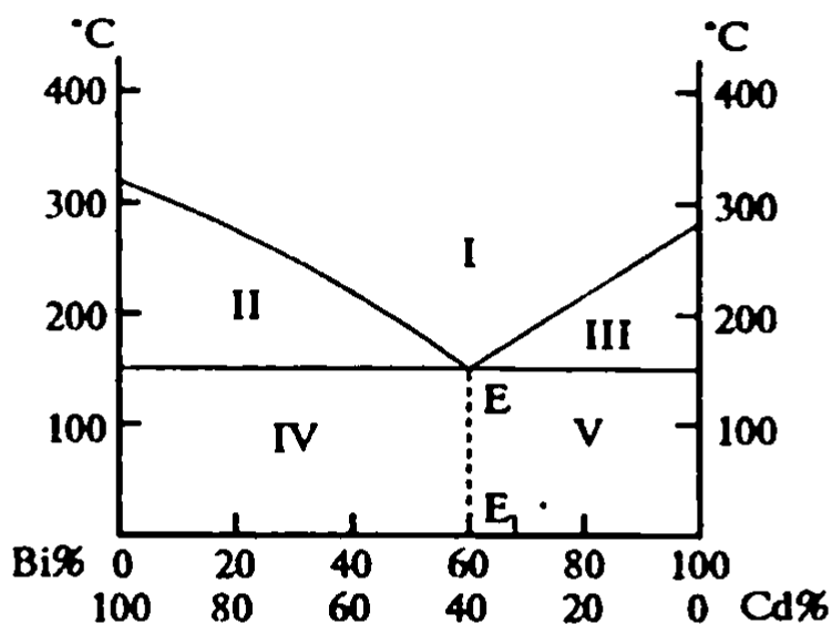
VIII.3-расм. Висмут-кадмий системасининг ҳолат диаграммаси.
