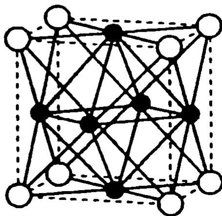
XI.6-расм. Олти ўзакли [Mo 6 Cl 4 ] 4+ катионининг тузилиши.
