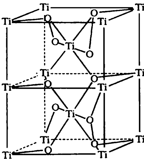
VI.3.-расм. Кўрғошин(IV) оксид билан бир хил тузилишга эга бўлган рутилнинг кристалл панжараси тузилиши.
