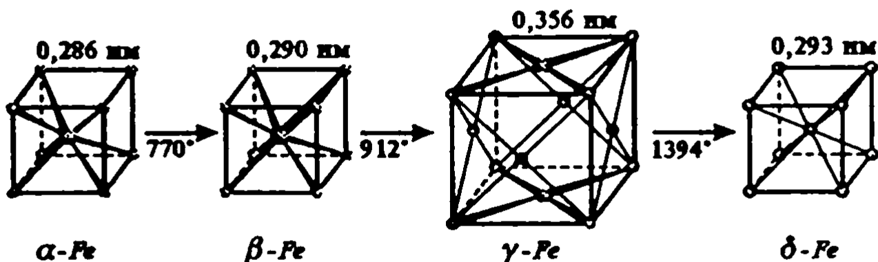
ХII.4-расм. Темирнинг полиморф шакли кўринишлари.
