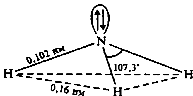
V.2-расм Аммиак молекуласининг тузилиши.
