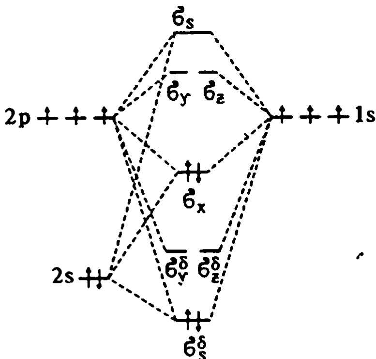
V.4-расм. Аммиак молекуласининг соддалаштирилган молекуляр орбиталар диаграммаси.
