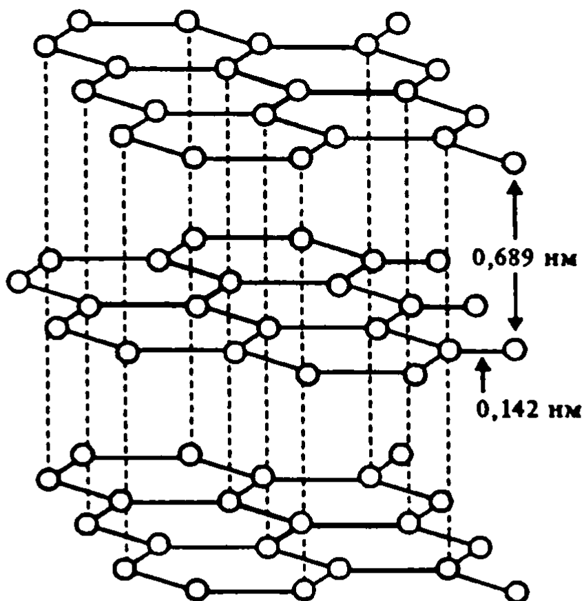
VI.2-расм. Графитнинг кристалл тузилиши.
