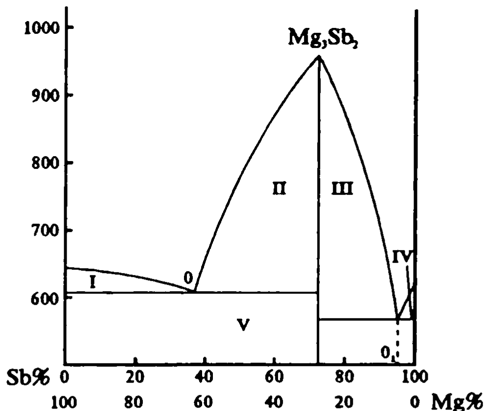
III.4-расм. Сурьма-магний системасининг ҳолат диаграмаси.
