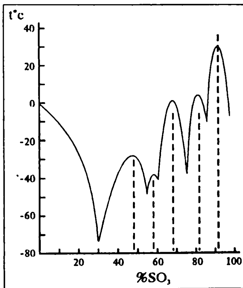
IV.2-расм. H_2O-SO_3 системасининг фазалар диаграммаси
