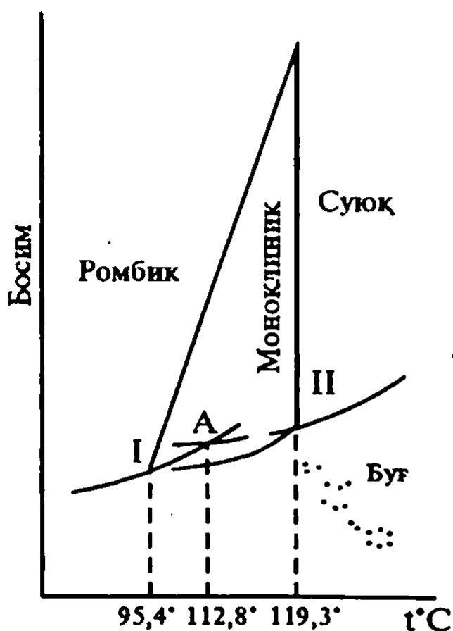
IV.1-расм. Олтингургуртнинг ҳолат диаграммаси.
