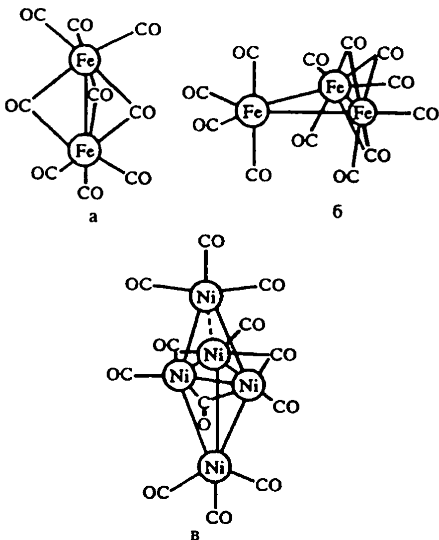
XII.7-расм. \text{Fe}_2(\text{CO})_9 (а), \text{Fe}_3(\text{CO})_{12} (б) ва \{\text{Ni}_5(\text{CO})_{12}\}^{2-} карбонилларнинг тузилиши.
