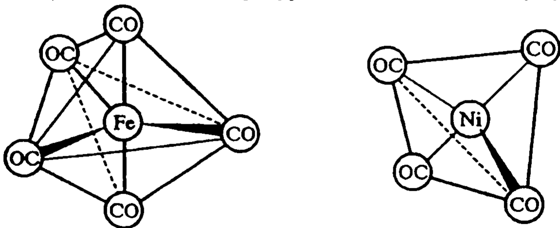
ХII.6-расм. \text{Fe}(\text{CO})_5 ва \text{Ni}(\text{CO})_4 ларнинг тузилиши.
