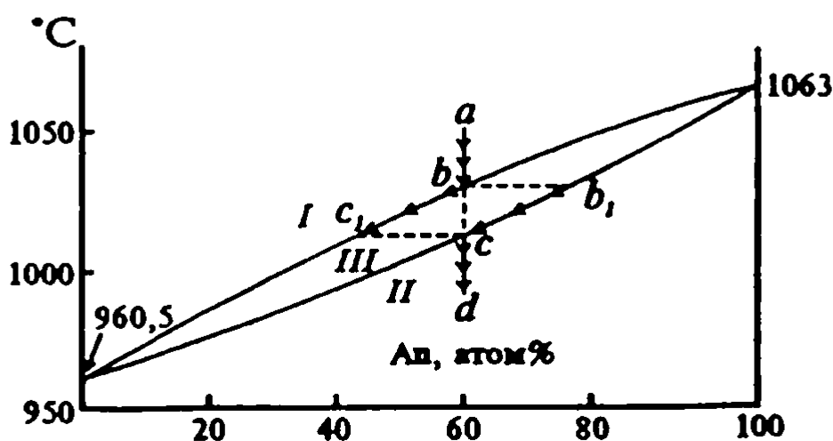
VIII.5-расм. Кумуш-олтин системасининг ҳолат диаграммаси.
