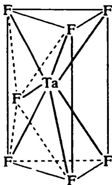
XII.1-расм. [TaF_7]^{2-} анионнинг тузилиши.
