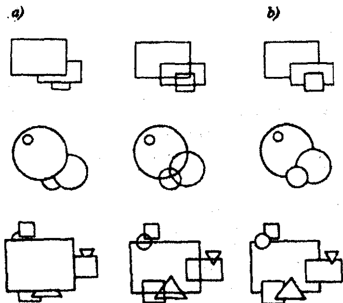
10-rasm. Belgilarni geometrik chizish uslubi: a – noto'g'ri, b- to'g'ri qurilgan.
