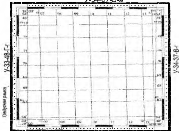
2.3-rasm. Topografik xarita ramkasi va ramka tashqarisidagi yozuvlar
