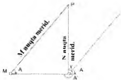
1.7.-rasm. Oriyentirlash burchaklari o'rtasidagi munosabat
