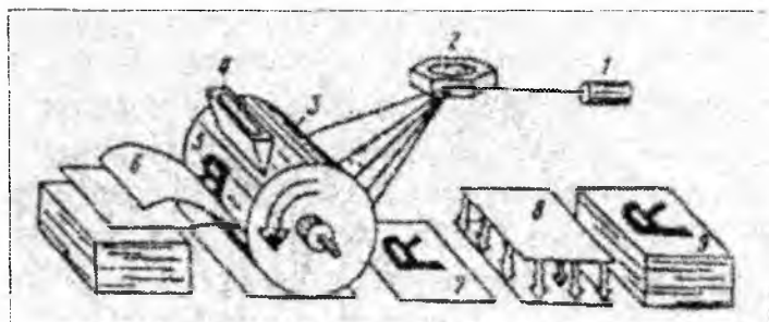
22.13-rasm. Elektronografik (lazer) printyerlarning ishlash chizmasi.
