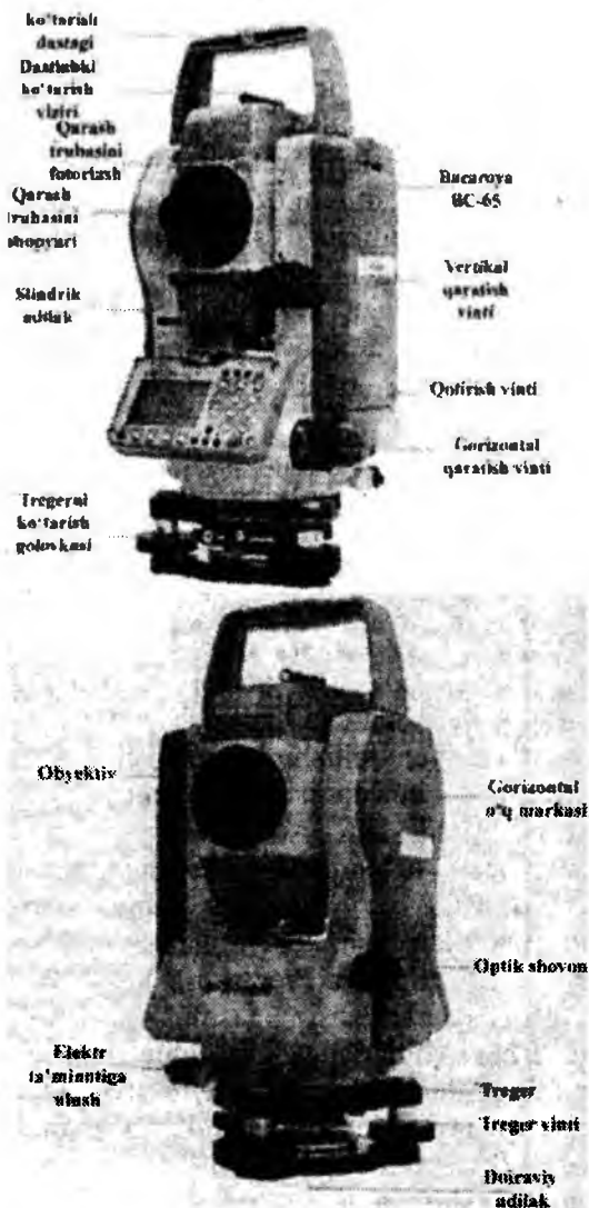
6.13-rasm. Elektron taxometr
