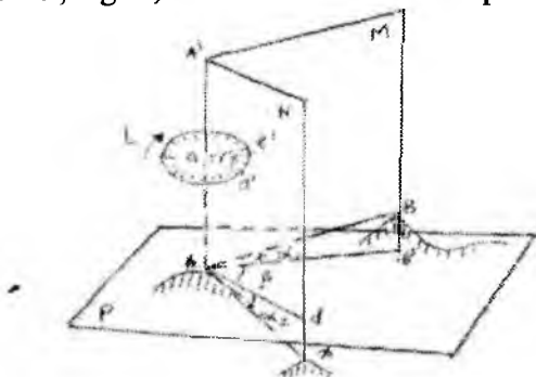
4.1-rasm. Gorizontol burchak oʻlchash sxemasi
