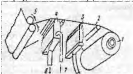
22.12-rasm. Elektrostatik bosma uskunaning ishlash chizmasi. 1-qog'oz ruloni, 2-qog'oz tasma, 3-elektrodlar, 4-bo'yovchi eritma, 5-qog'oz uzatish moslamasi, 6-ortiqcha bo'yoqning oqovasi, 7-bo'yoq berish moslamasi
