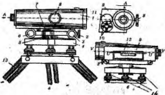
6.6-rasm. H3 niveliri tuzilishi
