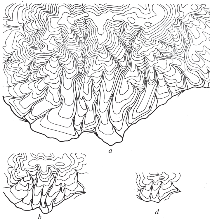
6.2-rasm. Gorizontallar usuli bilan tasvirlangan relifni masshtab asosida generalizatsiya qilish
