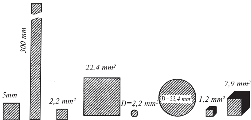
3.17-rasm. Bir xil o'lchamlar o'zaro nisbatini tavsiflovchi turli diagrammalar: chiziqli (ustunli); maydonli; hajmli.
