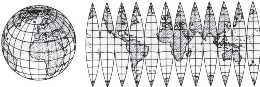
2.3-rasm. Meridianlar bo'yicha zonalarga (tilimlarga) bo'lingan globus yuzasi. Yerning egri yuzasini tekislikda uzilishsiz tasvirlab bo'lmagligini tasdiqlovchi sxema.
