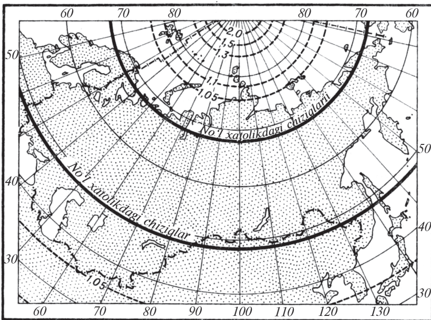
2.13-rasm. Kavrayskiyning teng oraliqli konusli proyeksiyasida kartografik to'ra.
