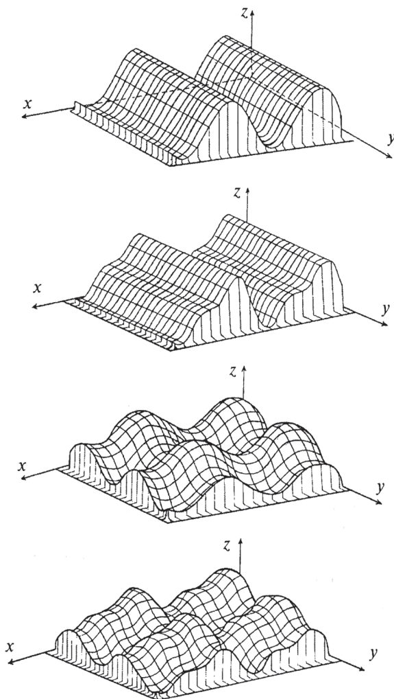
12.16-rasm. Ikki o'lchamli sinusoidal to'liqlarni bir-biriga ketma-ket joylashtirish yordamida hosil bo'lgan yuzaning trigonometrik approximationsiyasi chizmasi.
