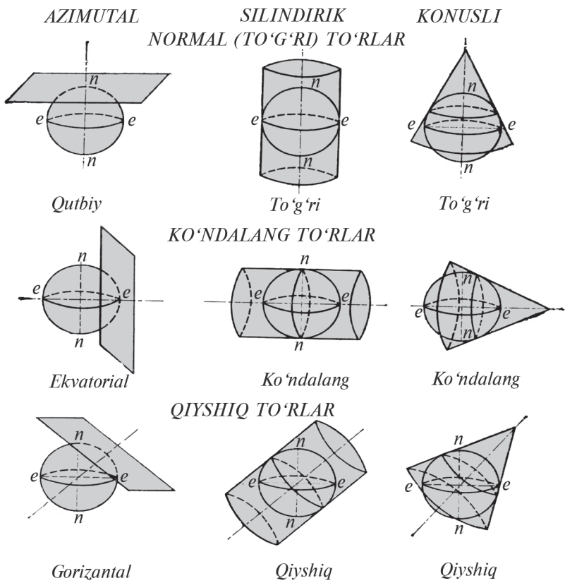
2.8-rasm. Yordamchi geometrik yuzalarni oriyentirlash.
