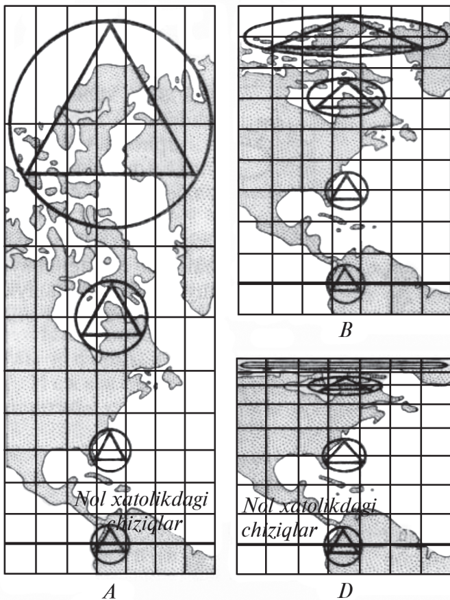
2.6-rasm. Silindrik proyeksiyalarda tuzilgan kartalardagi xatoliklar ellipsi: A – teng burchakli; B – teng maydonli (yoki ekvivalent); D – ixtiyoriy (teng oralikli). Xatoliklar ko‘rgazmali bo‘lishi uchun aylana ichiga teng tomonli uchburchak chizilgan.
