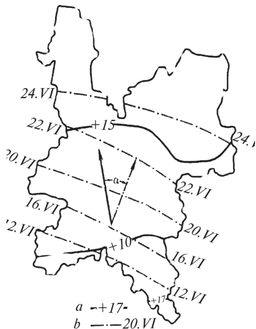
12.19-rasm. Yuzalarning eng katta qiyaligi kosinus burchagi bo'yicha taqribiy korrelyasiya koeffitsientini aniqlash.
