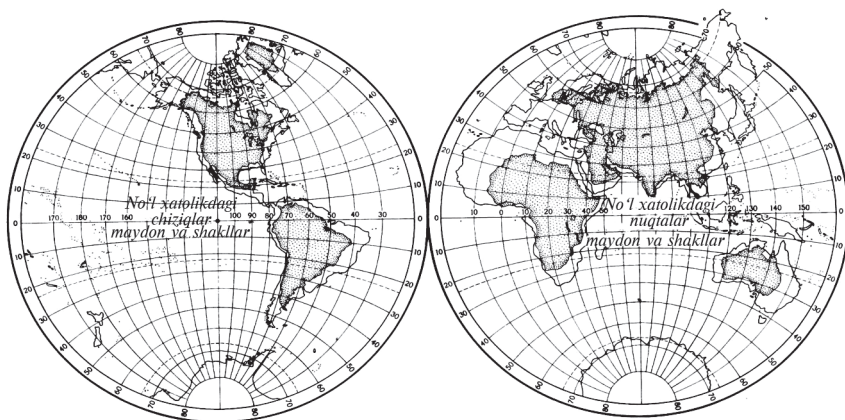
2.11-rasm. Sharqiy va gʻarbiy yarim sharlarning koʻndalang azimutal stereografik proyeksiyada tuzilgan kartalari.
