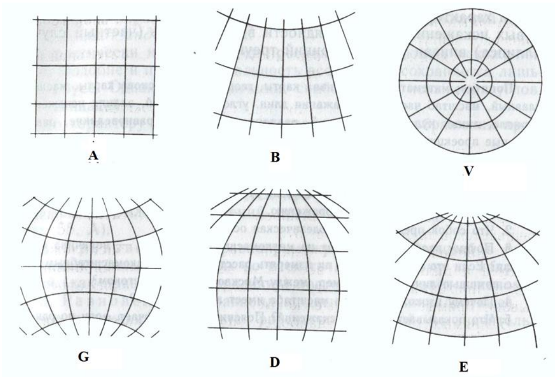
8.7-rasm. Normal (to'g'ri) proyeksiyalarda meridian va parallellarni ko'rinishi: A – slindrik; B – konusli; V – azimutal; G – ko'pkonusli; D – psevdoslindrik; E – psevdokonusli
