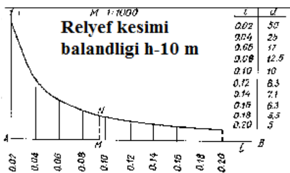
3.4-rasm. Nishablik mashtabi grafigi
