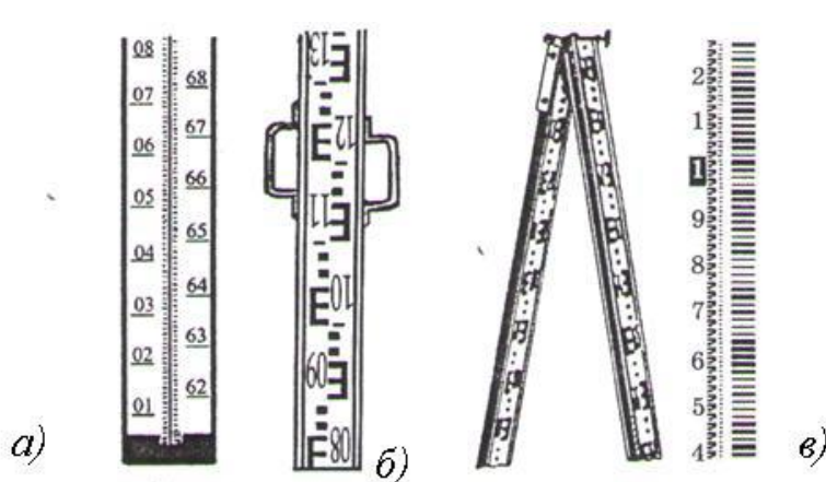
6.9-rasm. Nivelirlash reykalari
