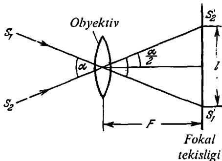
61-rasm. Fotografik tasvirning chiziqli o'lchami
