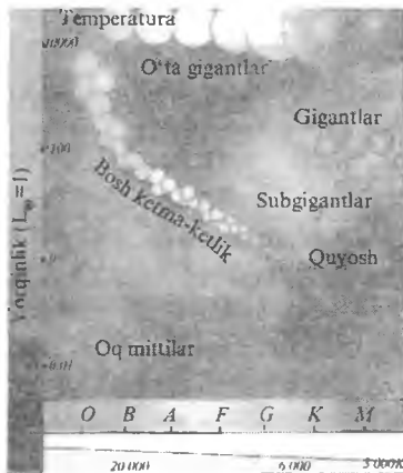
Spektral sinflar va temperatura
