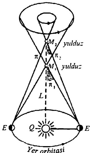
120-rasm. Yulduzning yillik parallaksi va unigacha masofani aniqlash usuli
