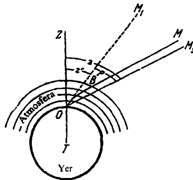
18-rasm. Astronomik refraksiya hodisasi
