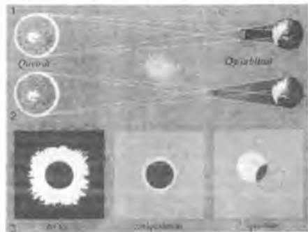
47-rasm. Quyoshning to'la, halqasimon va qisman tutilishi chizmasi
