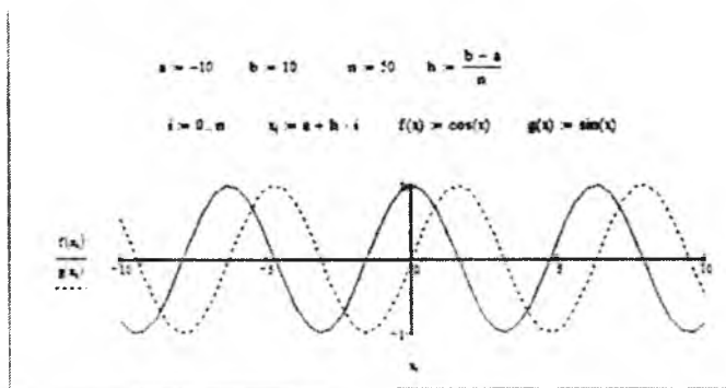
11.14-rasm. \cos(x) va \sin(x) grafigi.
