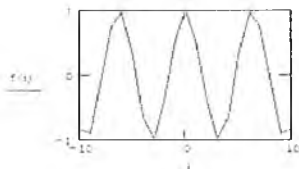
11.13-rasm. \cos(x) grafigi.
