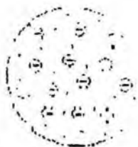
Модель У. Томсона. 1902 г.
