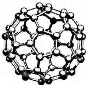
43-rasm. Fulleren molekulası
