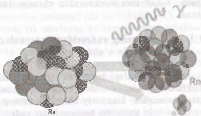
\alpha - parchalanish animatsiyasi.
