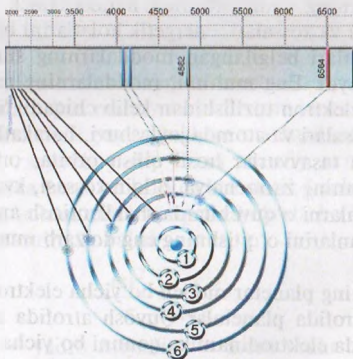
Vodorod atomining ko'rinadigan spektri.
