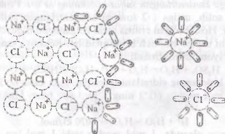
Natriy xloridning suvdagi eritmasida elektrolitik dissotsiatsiyalanishi.
