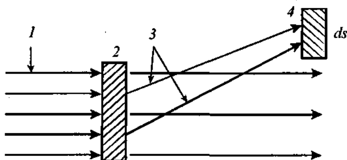
5.4-rasm. Yadro reaksiyasini o'rganishga doir tajriba sxemasi. 1 — tushayotgan \alpha -zarralar; 2 — nishon yadro; 3 — reaksiya natijasida hosil bo'lgan yadro; 4 — detektor.
