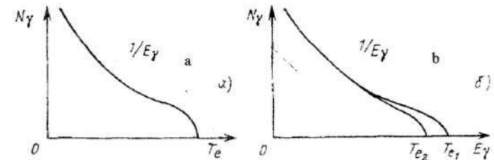
5.3-rasm. Tormozli nurlar spektrini: a-energiyasi T_e bo‘lgan elektronlar hosil qilgan spektr; b-energiyalari T_{e1} va T_{e2} bo‘lgan elektronlar hosil qilgan spektrlar.
