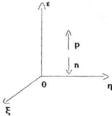
2.2-rasm. Izotopik spin.
