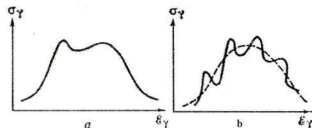
5-rasm. Gigant dipol rezonansining nozik strukturasi: a–deformatsiyalangan yadrolar uchun; b–sferik yadrolar uchun
