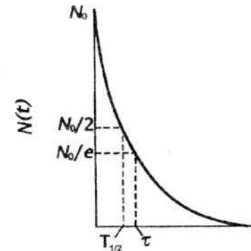
4.2-rasm. Radioaktiv parchalanishning eksponensial qonuni. Parchalanmagan yadrolar soni vaqt o'tishi bilan eksponenta bo'yicha kamayadi. Bu yerda yarim parchalanish davri T_{1/2} va o'rtacha yashash vaqti \tau = 1/\lambda keltirilgan.
