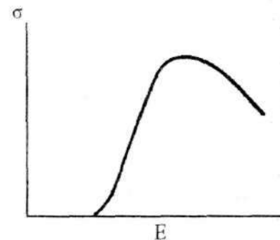
5.7-rasm. Reaksiya kesimining zaryadlangan zarra energiyasiga bog'lanishi.
