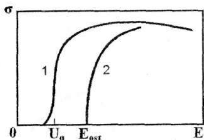
5.8-rasm. Ekzotermik va endotermik yadro reaksiyalarining uyg'onish funksiyalari.
