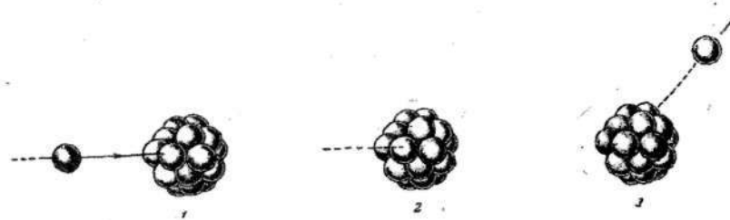
5.1-rasm. Oraliq yadro mexanizmining yuz berish bosqichlari.
