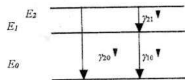
4.7-rasm. \gamma - o'tishlar sxemasi.
