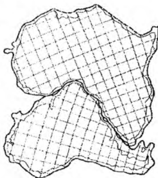
12.4-rasm. Janubiy Amerika va Afrika materiklari chegaralarini 200 m izobata bo'yicha birlashtirish.
