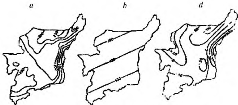
13.4-rasm. Issiq davrda yog'in-sochin miqdori kartasi (a), approssimasiyadan keyingi fonli (b) va qoldiq (d) yuzalar
