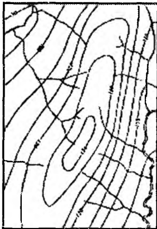
13.5-rasm. Soddashtirish. Zamonaviy relief kartasini morfo-izogips kartasiga aylantirish: a – zamonaviy relief; b – umumlashgan gorizontallar yordamida reliefni tasvirlash.
