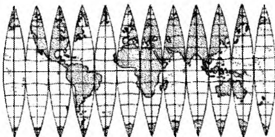
2.3-rasm. Meridianlar bo'yicha zonalarga (tilimlarga) bo'lingan globus yuzasi. Yerning egri yuzasini tekislikda uzilishsiz tasvirlab bo'lmagligini tasdiqlovchi sxema.
