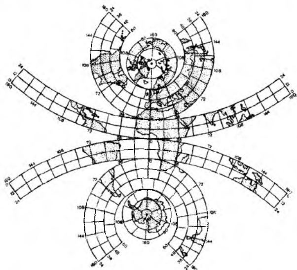
9.1-rasm. 1:2 500 000 mashtabli dunyo kartasi razgrafkasi.
