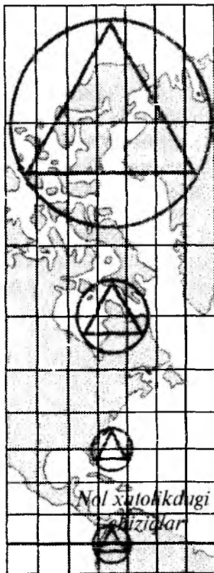
2.6-rasm. Silindrik proyeksiyalarda tuzilgan kartalardagi xatoliklar ellipsi: A – teng burchakli; B – teng maydonli (yoki ekvivalent); D – ixtiyoriy (teng oraliqli). Xatoliklar ko'rgazmali bo'lishi uchun aylana ichiga teng tomonli uchburchak chizilgan.
