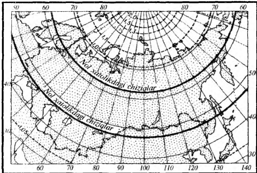
2.14-rasm. Krasovskiyning teng oraliqli konusli proyeksiyasida kartografik to'ra.
