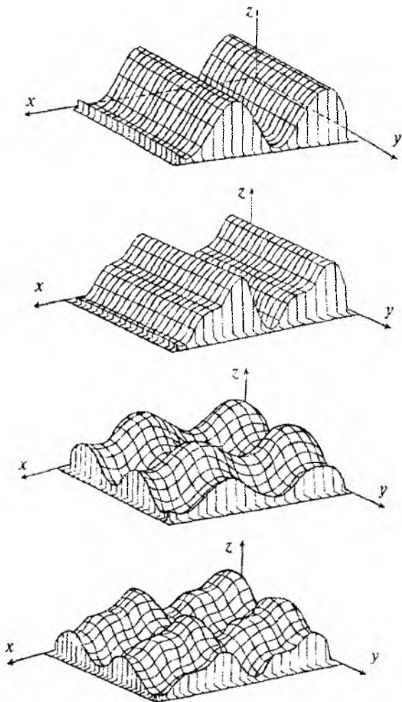
12.16-rasm. Ikki o'ichamli sinusoidal to'liqlarni bir-biriga ketma-ket joylashtirish yordamida hosil bo'lgan yuzaning trigonometrik approksimatsiyasi chizmasi.
