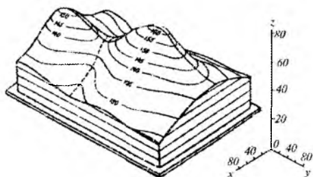
12.9-rasm. Vertikal bo'yicha turli mashtabga ega bo'lgan blok-diagramma.
