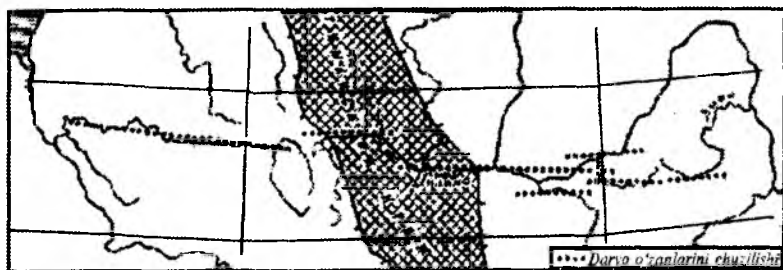
13.2-rasm. Nuqtalar bilan daryo o'zganlarining cho'zilishi berilgan.
