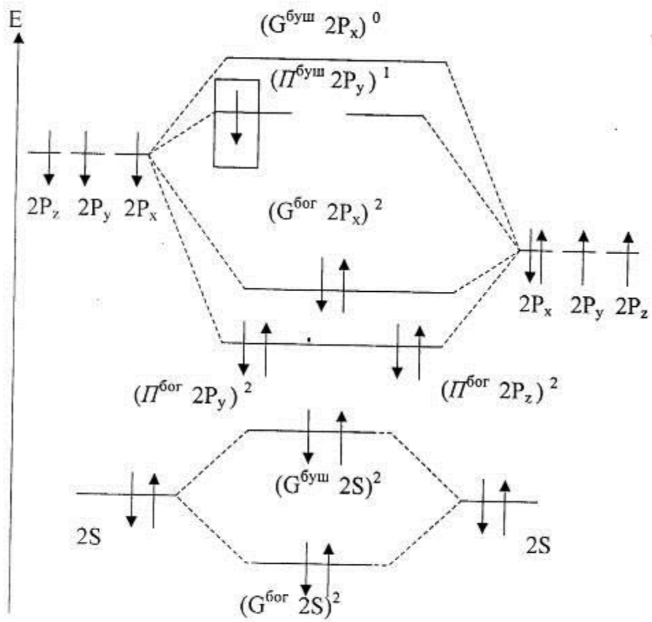
9-Расм NO + ионининг ҳосил булиш МО лари энергетик диаграммаси
