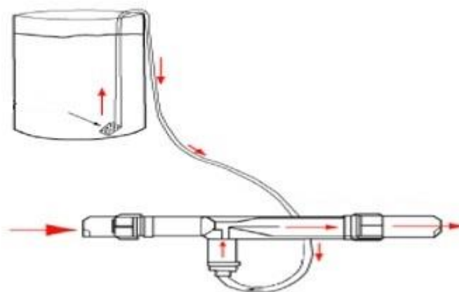
2.9.12-rasm. Venturi o'g'itlash purkagich uskunasi.
