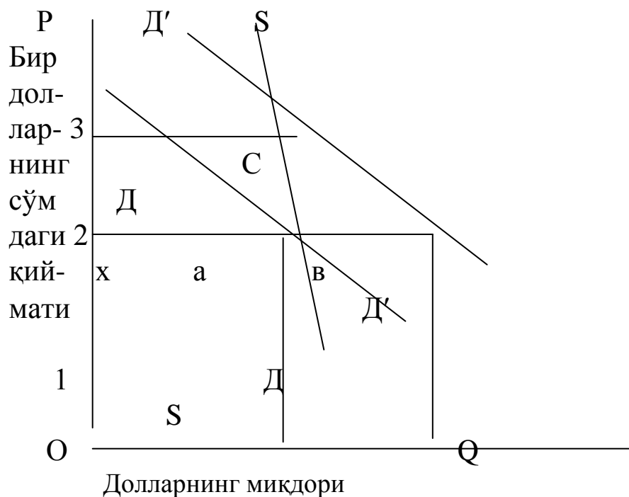
3.8.4-чизма. Эгилувчан валюта курлари шароитидаги тенглик.
