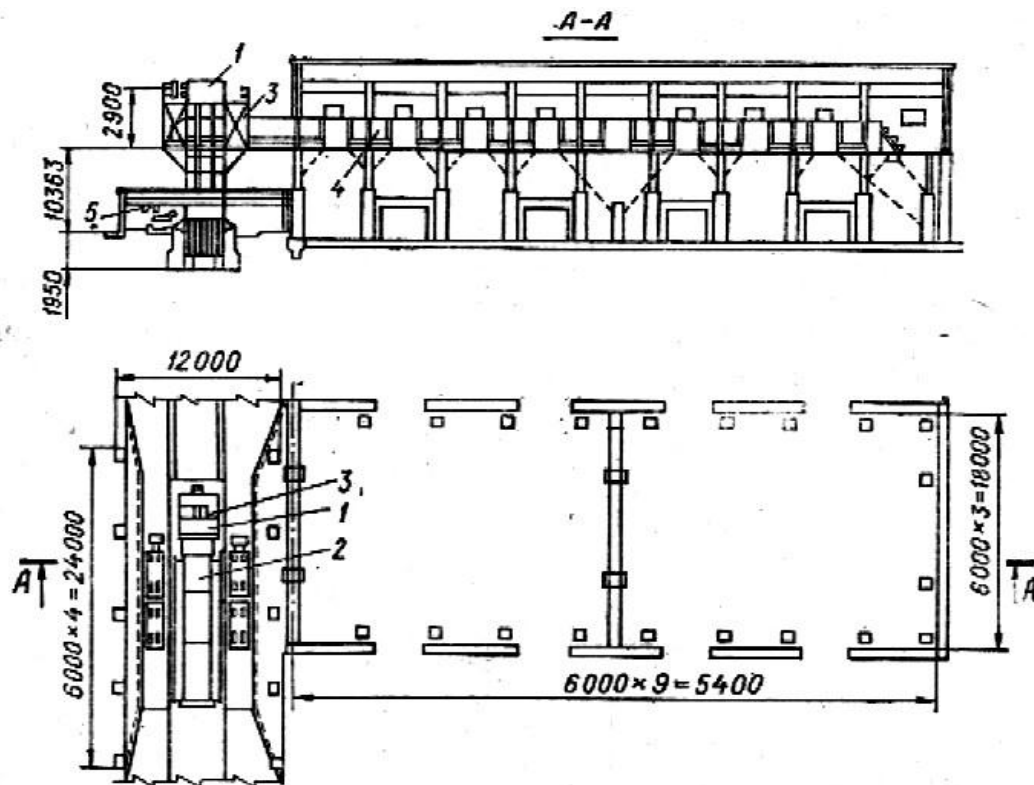
1-chizma. 700 t paxta saqlash uchun mexanizatsiyalashtirilgan yopiq ombor sxemasi:
