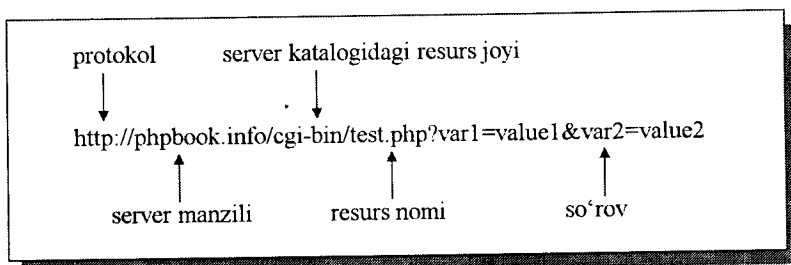
4.1-rasm. URLning to'liq shakli.
