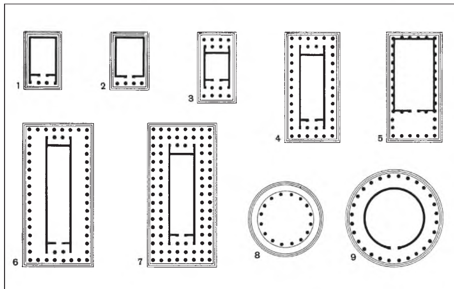
Типы греческих храмов.
