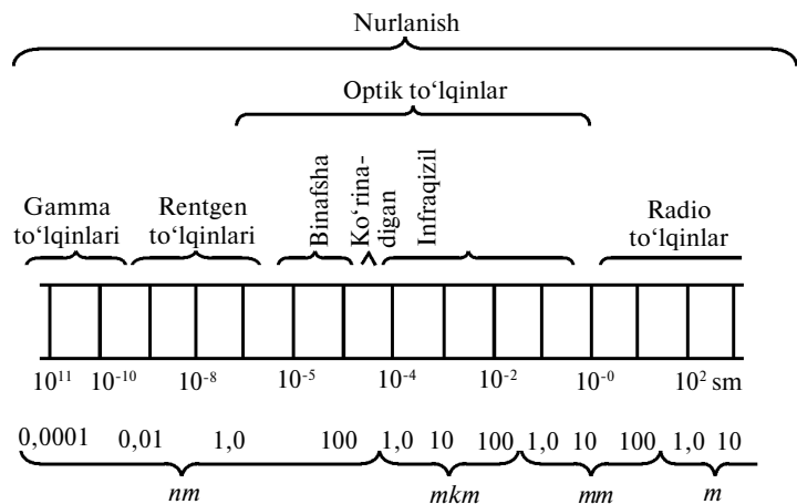
59-rasm. Aerokosmik syomkadan foydalaniladigan elektromagnit to'liqinlar spektri.
